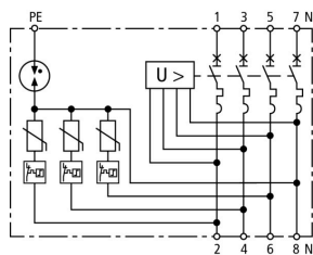
Prinzip Schaltbild SPD+POP 4 255 C63
