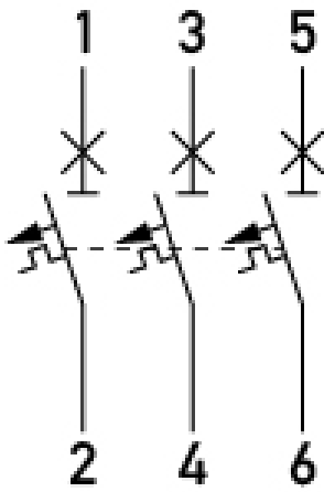
Anschlusschema
