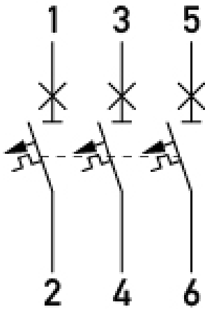
Anschlusschema
