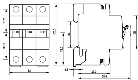
Maßzeichnung Gruppenansicht
