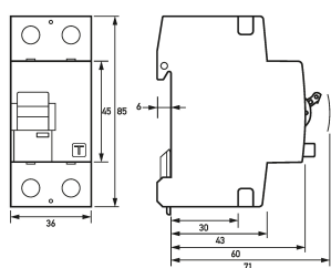
Maßzeichnung Gruppenansicht
