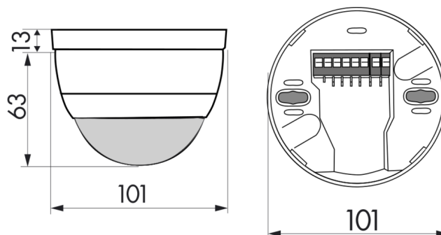
Bemaßung 92440
