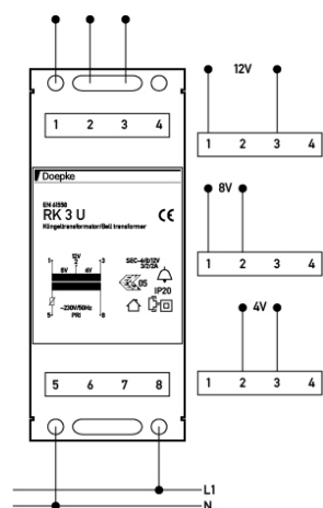
Anschlusschema
