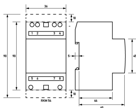
Maßzeichnung Gruppenansicht
