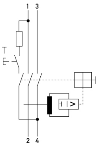
Anschlusschema
